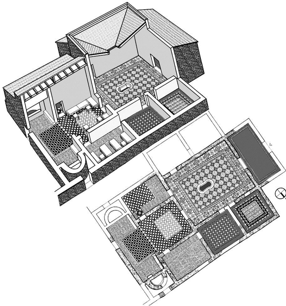
Сл. 2 Стакина чешма, Валандово, приградска вила, реконструирана основа и перспектива (4 век н.е.)
